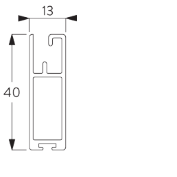
SG 10993 Bottom bar
