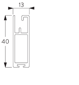
SG 10993 Bottom bar
